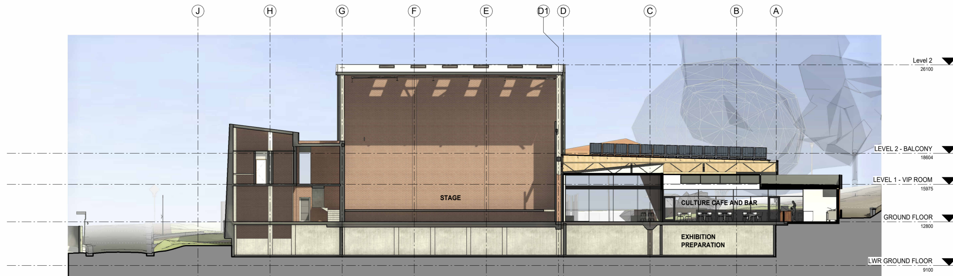
E SECTION E-E 1 : 200
