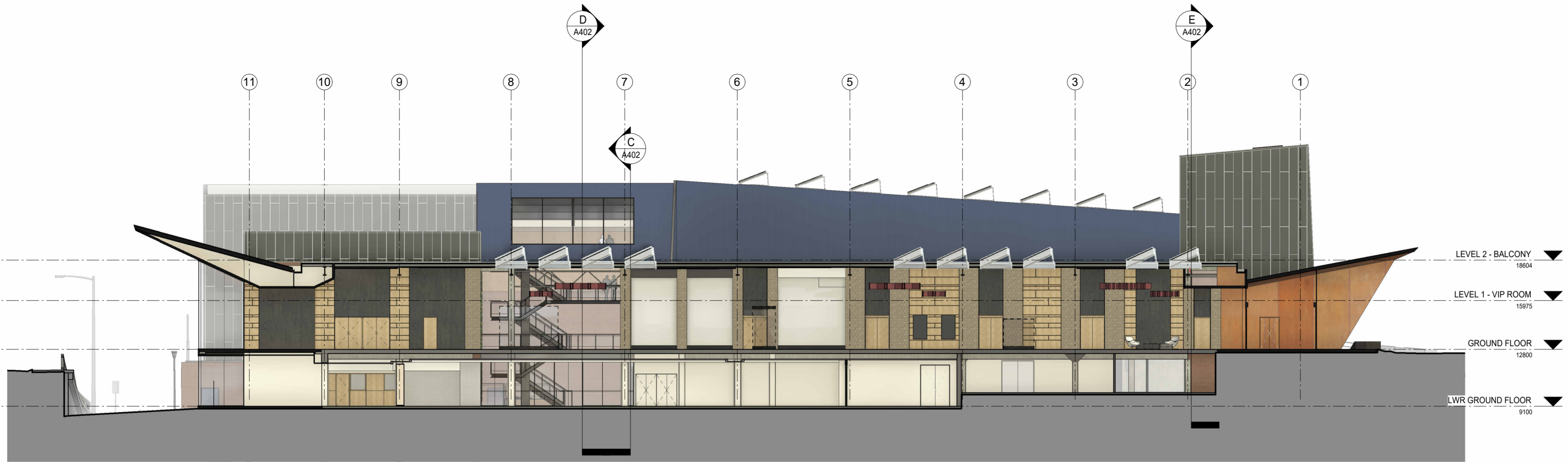
A SECTION A-A 1 : 200
