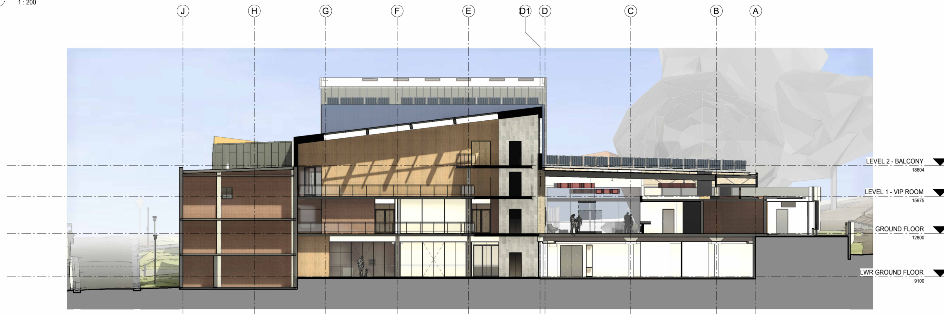
D SECTION D-D 1 : 200
