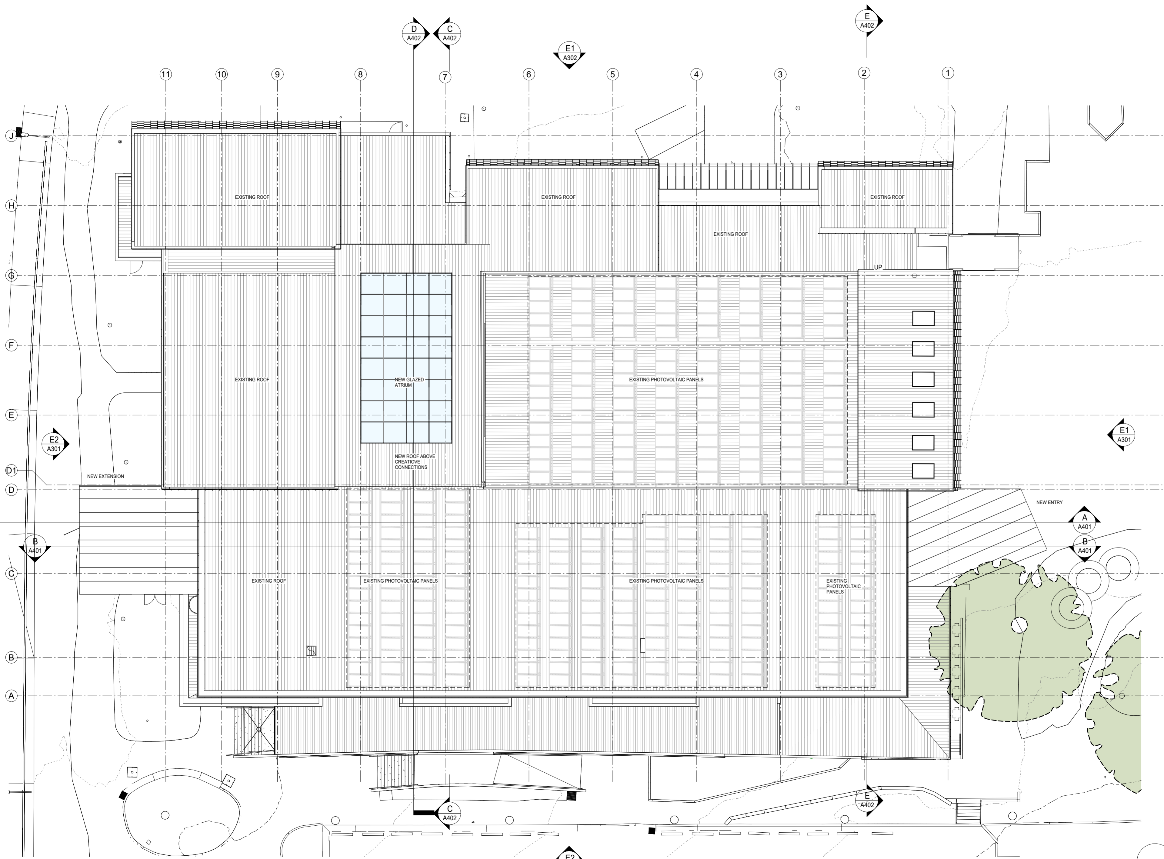
1 ROOF PLAN 1 : 200
